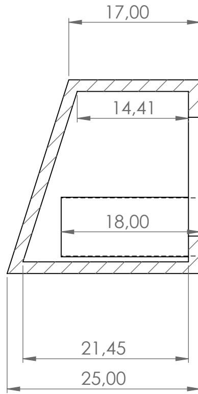
SEÇÃO D-D
