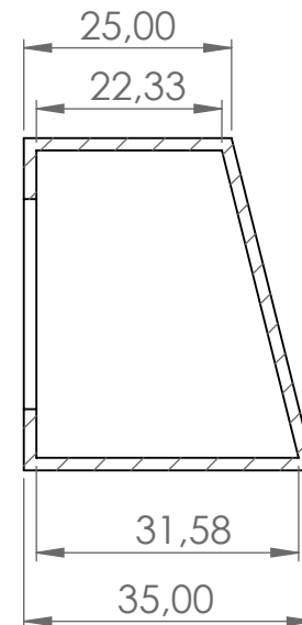
SEÇÃO F-F ESCALA 1 : 1
