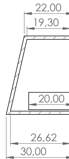
SEÇÃO E-E ESCALA 1 : 1
